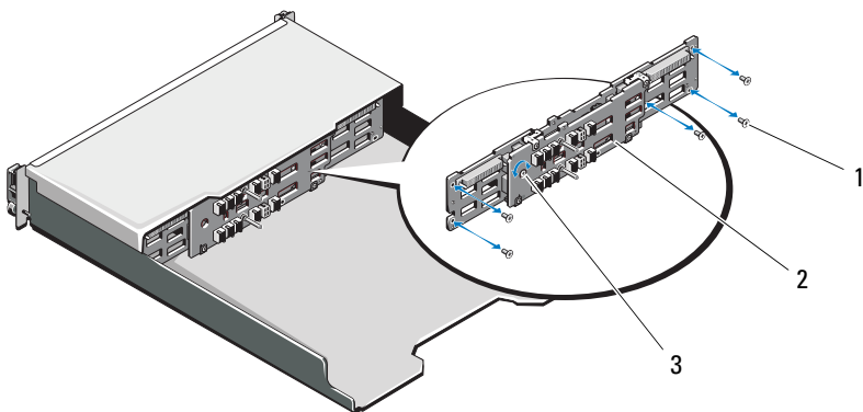
图 16-16. 卸下和安装背板 -PowerVault MD3600f
